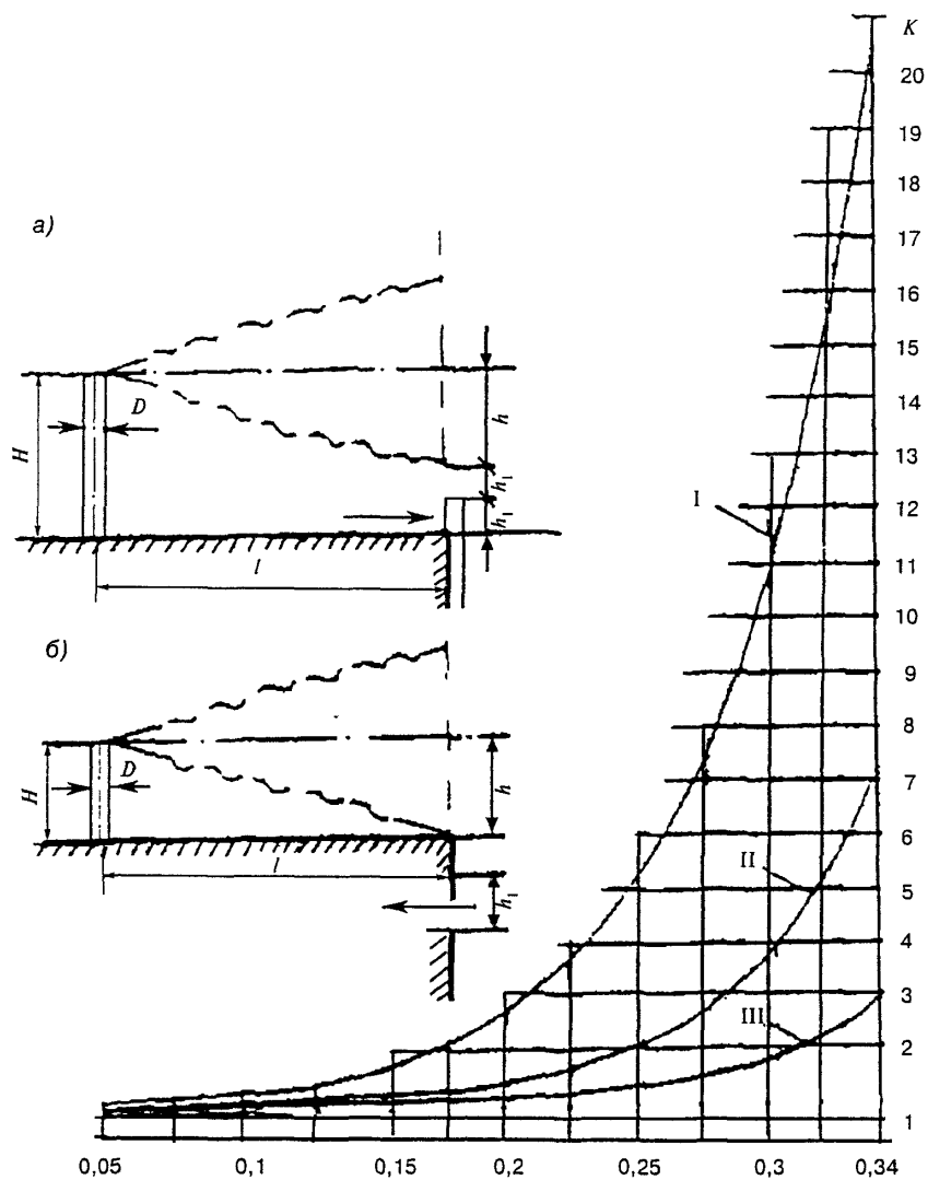
а - расположение источника над зоной всасывания наружного воздуха приемным устройством (высота трубы источника H = 2h_1 + h ); б - то же, над кровлей здания (высота трубы источника H = h ); h - расстояние по вертикали, м, горизонтальной оси струи; h_1 - высота отверстия для приема наружного воздуха, м; l - расстояние между устьем источника и приемным устройством для наружного воздуха, м
